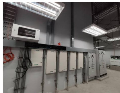
งานติดตั้งตู้ไฟฟ้าคอนโทรล
