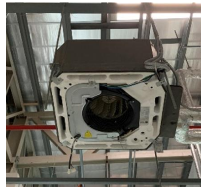
งานติดตั้งเครื่องส่งลมขนาดเล็ก
